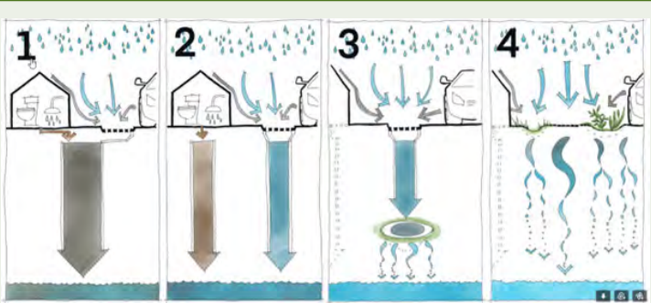
Myndin sýnir fjórar byltingar í meðferð ofanvatns. Innleiðing blágrænna innviða tryggir náttúrulega hreinsun ofanvatns með jarðvegi og gróðri, um leið og dregið er úr álagstoppum á veitukerfi. Mynd / Herborgdraws.com, Alta
